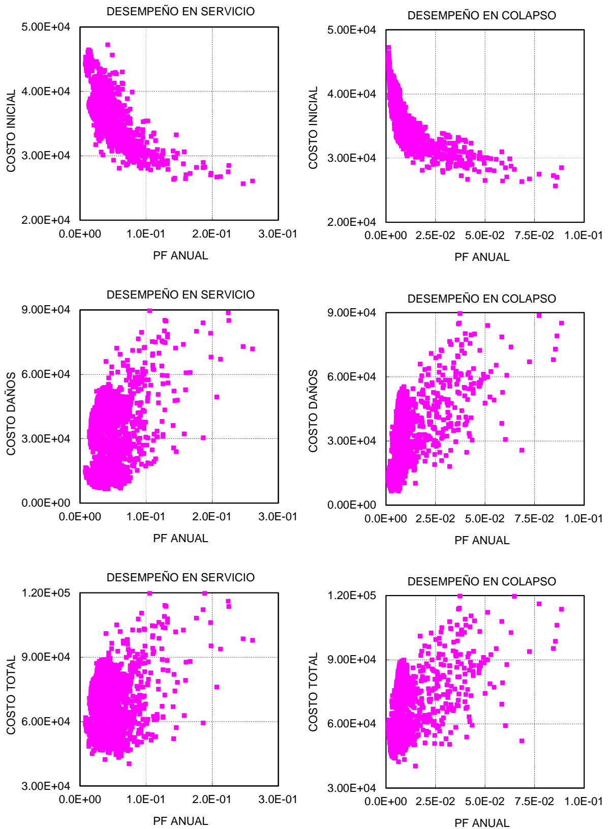
Figura 6: Frente Pareto y probabilidad de falla óptima para \nu = 1
