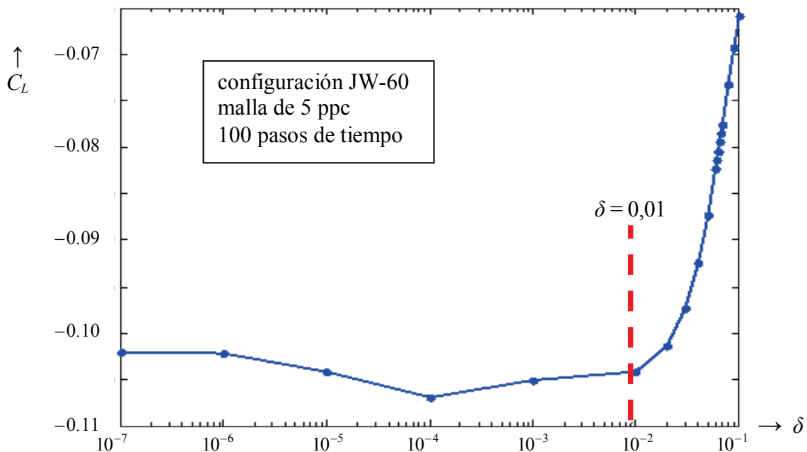
Figura 16: Variación de C_L en función del parámetro cutoff
