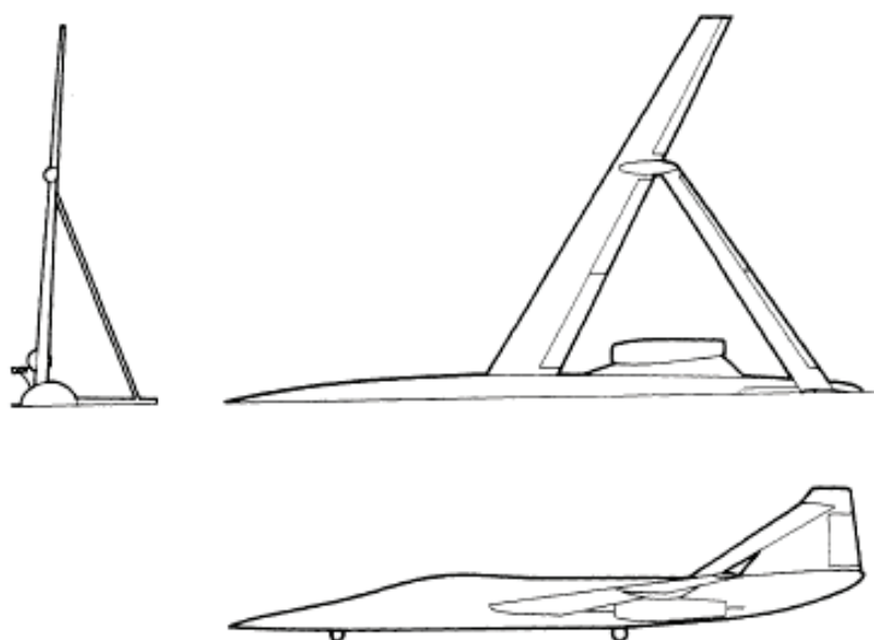
Figura 2: Diseño conceptual del avión JWRA (Smith y Stonum, 1989)
