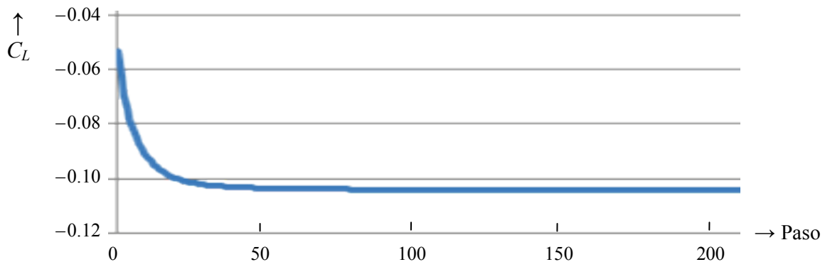
Figura 15: C_L vs. paso de tiempo computacional para la configuración JW-60
