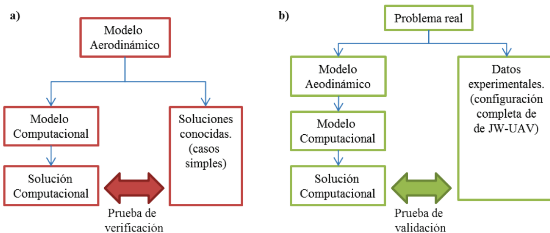
Figura 3: Esquematización de los procedimientos realizados. a) verificación y b) validación
