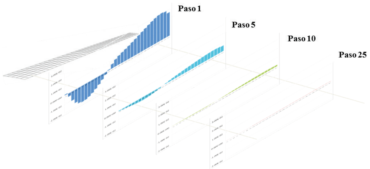
Figura 13: representación esquemática de la evolución de los valores de la circulación \Gamma en el borde de fuga del ala delantera de la configuración JW-60
