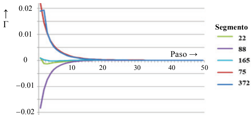
Figura 14: Evolucion temporal de \Gamma para algunos segmentos vorticosos del borde de fuga del ala delantera
