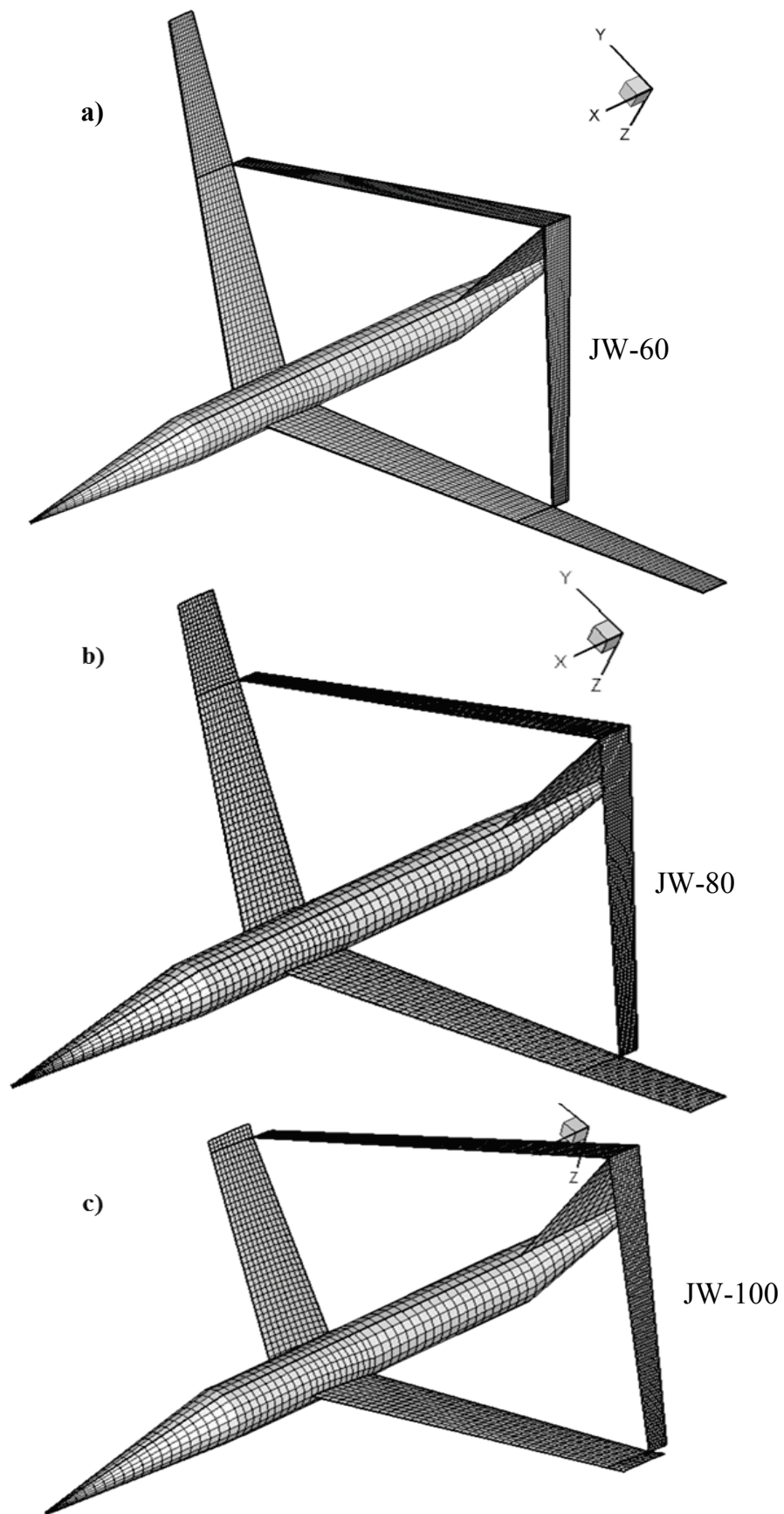
Figura 11: Modelo geométrico-computacional para las configuraciones: a) JW-60, b) JW-80 y c) JW-100
