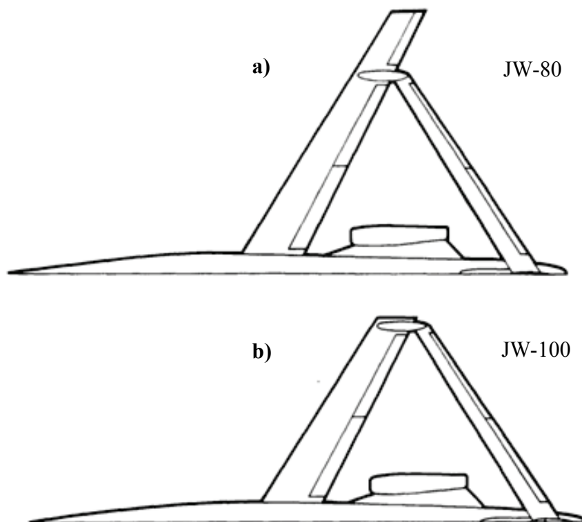
Figura 8: Avión de alas unidas denominado JWRA a) configuración JW-80 y b) configuración JW-100 (Smith y Stonum, 1989)
