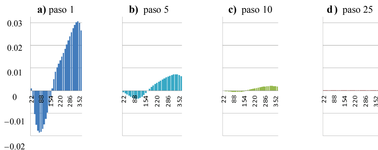
Figura 12: Valores de \Gamma de segmentos emisores de vorticidad del ala delantera, para los pasos de simulación: a) 1, b) 5, c) 10 y d) 25
