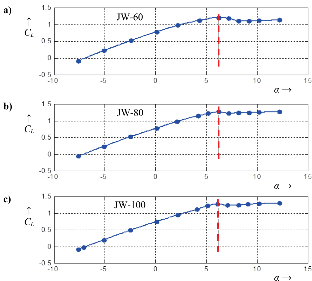
Figura 9: Curvas experimentales del coeficiente de sustentación C_L en función del ángulo de ataque \alpha para las configuraciones a) JW-60, b) JW-80 y c) JW-100 (Smith y Stonum, 1989)
