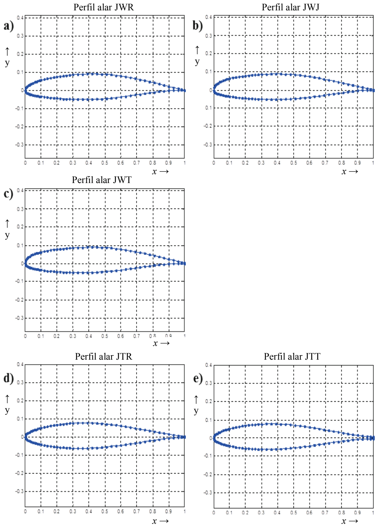
Figura 10: Datos geométricos de perfiles alares a) JWR, b) JWJ, c) JWT, d) JTR y e) JTT (Smith y Stonum, 1989)
