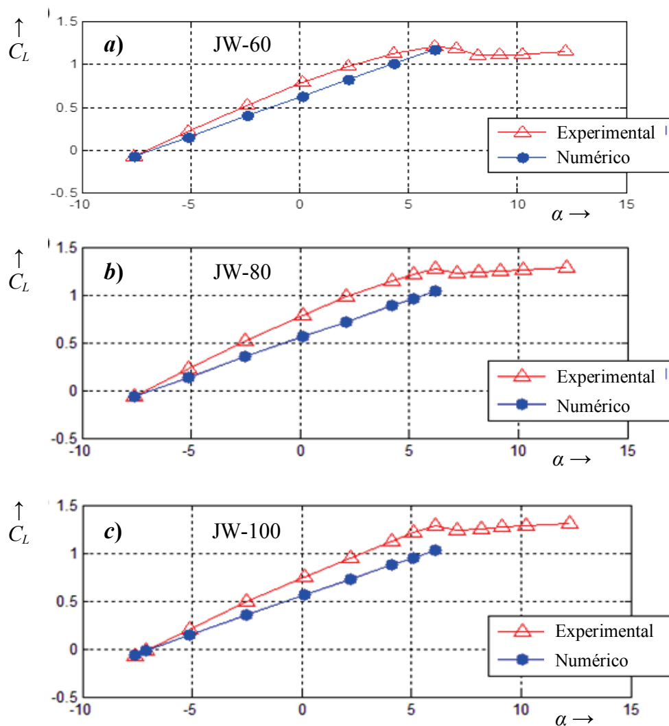
Figura 17: Comparación de resultados numéricos y experimentales del coeficiente de sustentación C_L
