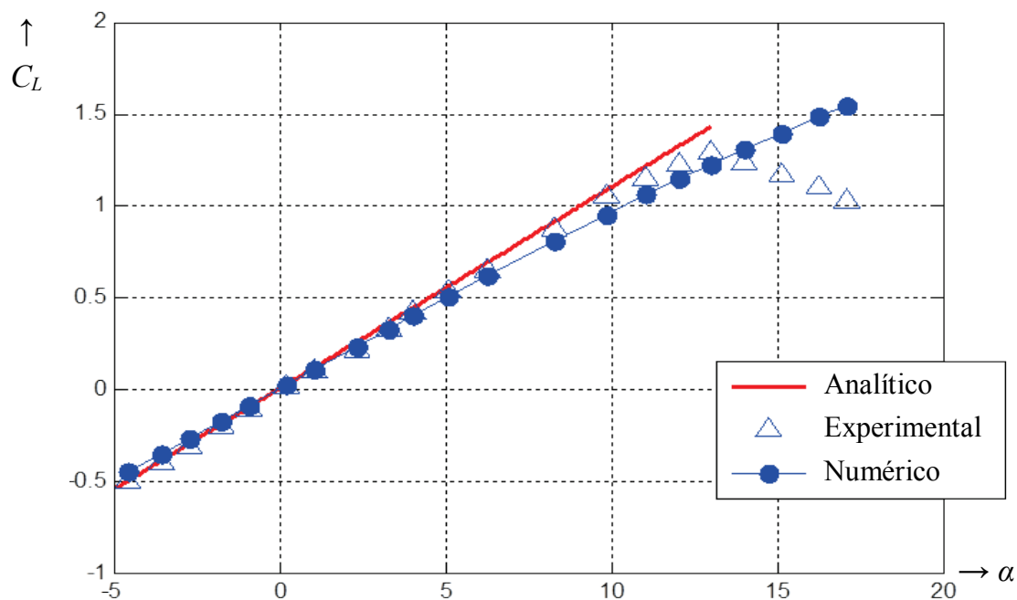
Figura 7: Variación del coeficiente de sustentación C_L en función del ángulo de ataque \alpha para un perfil NACA 0009
