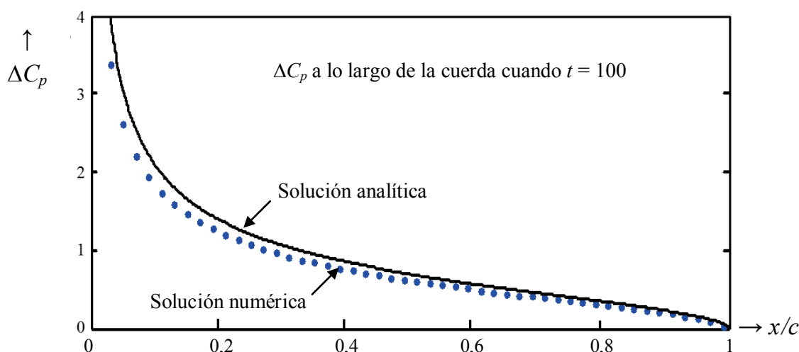
Figura 6: Distribución del salto del coeficiente de presión \Delta C_p a lo largo de la cuerda en el centro del ala
