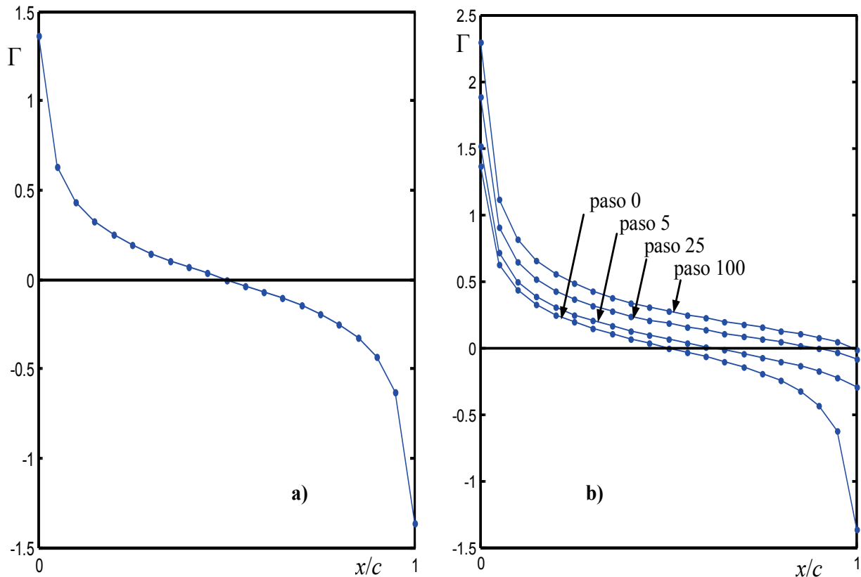
Figura 5: Circulación \Gamma a largo de la cuerda media de un ala de gran alargamiento. a) Paso de tiempo 0, b) evolución temporal (algunos pasos de tiempo)
