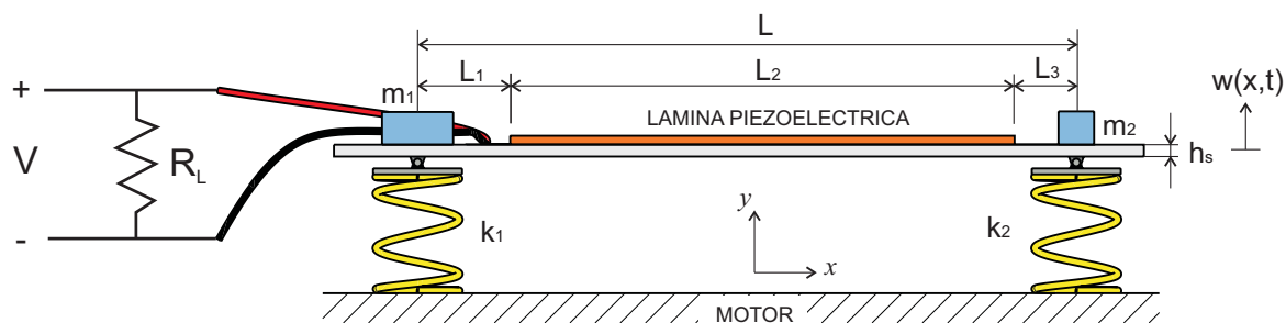
Figura 1: Esquema del dispositivo recolector
