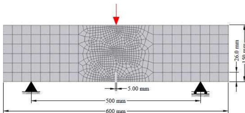
Figura 6: Malla de elementos finitos correspondiente a la viga entallada.
